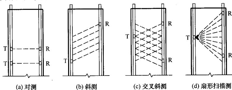
图 D.0.3-4 钻孔法示意图
