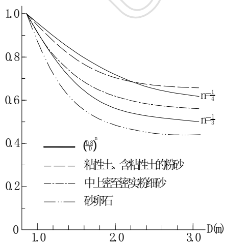
图 5.3-4 大直径桩端阻尺寸效应系数 \psi_p 与桩径 D 关系计算与试验比较
