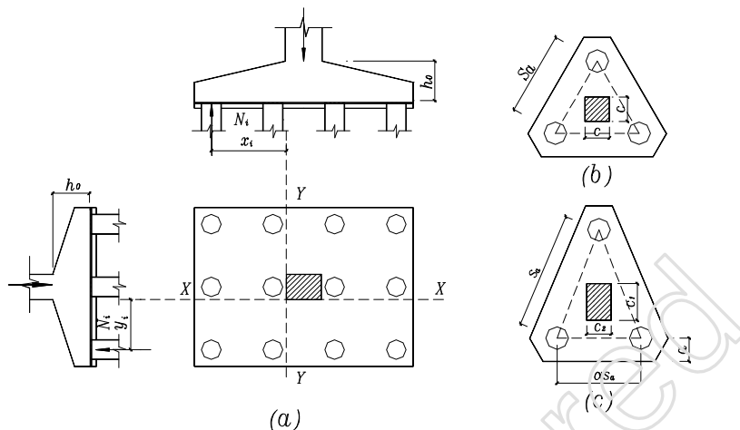
图 5.9.2 承台弯矩计算示意
