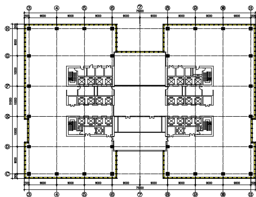
图 5.5-4 标准层平面图
