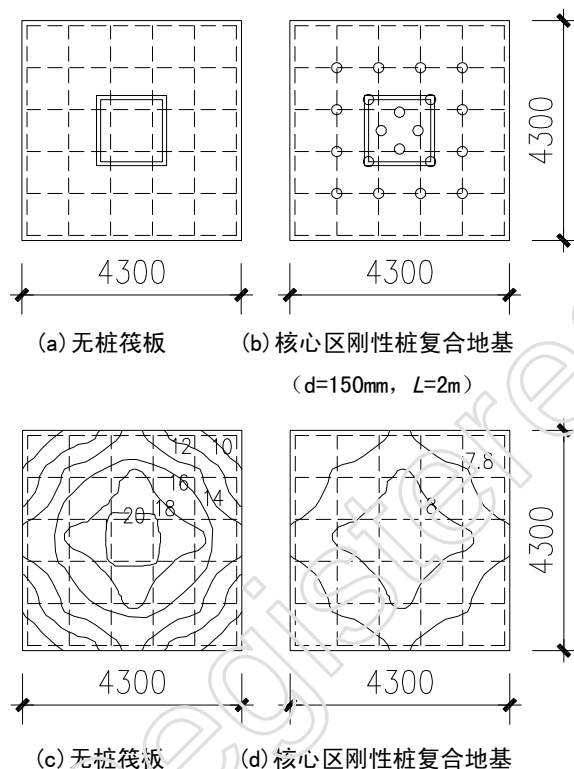
图 3.1-7 核心区局部增强(刚性桩复合地基)与无桩筏板模型试验 ( P=3250\text{kN} )
