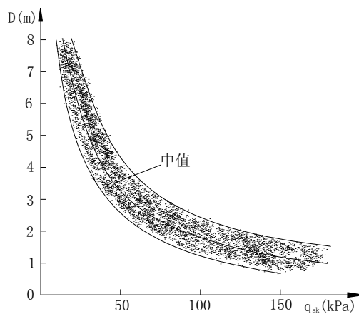
图 5.3-5 砂、砾土中极限侧阻力随桩径的变化
